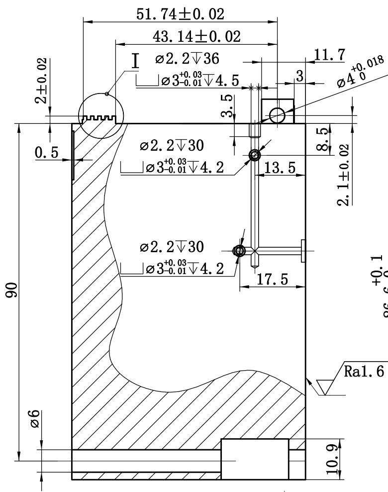
D向
