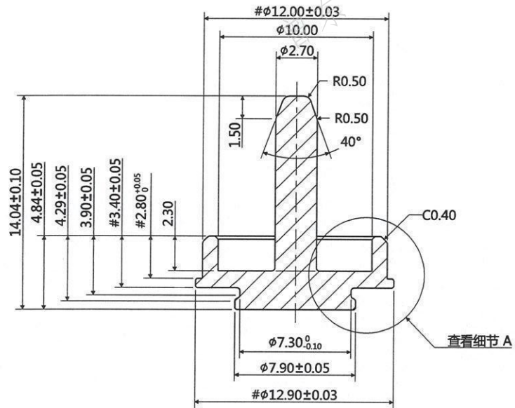
截面 A-A
