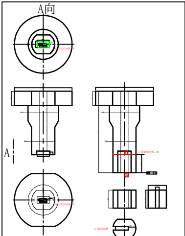
3.1 切断、割槽、钻螺栓孔、 3.2 螺纹孔，火花沉孔4mm
