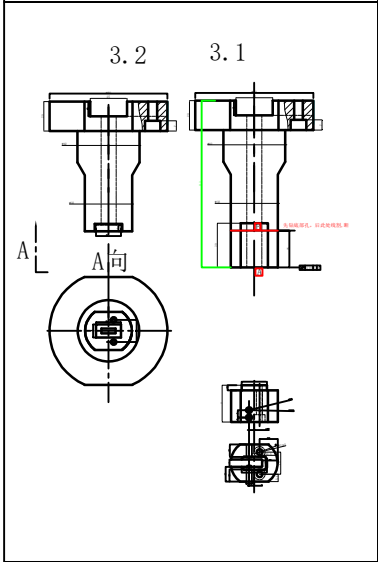
3.1 切断、割槽、钻螺栓孔、 3.2 螺纹孔，火花沉孔4mm
