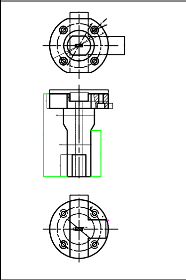
2. 针套铣T槽， 钻安装孔
