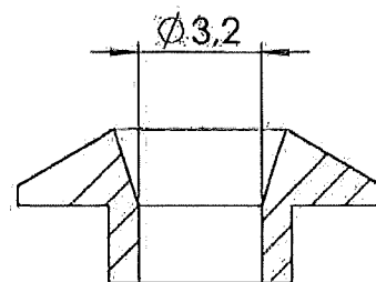
SCHNITT A-A
